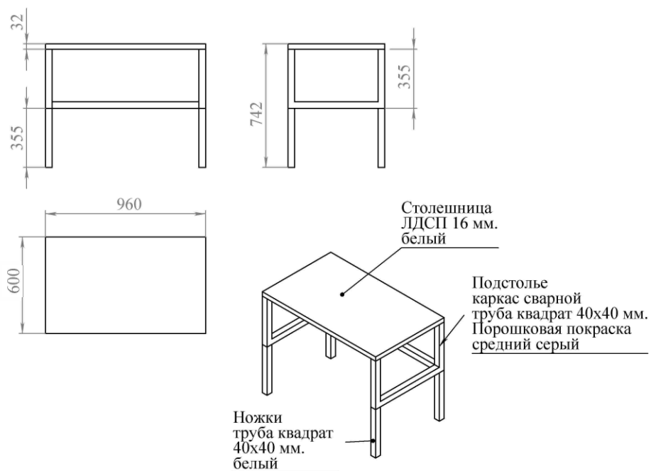
Стол ученический одноместный на сварном составном каркасном подстоле
