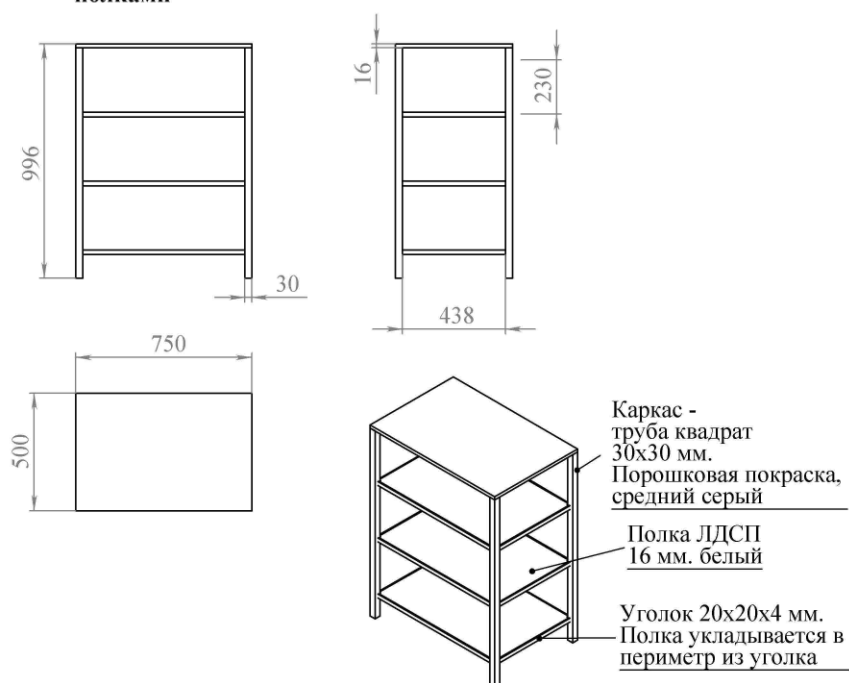
Каркас с внутренними полками
