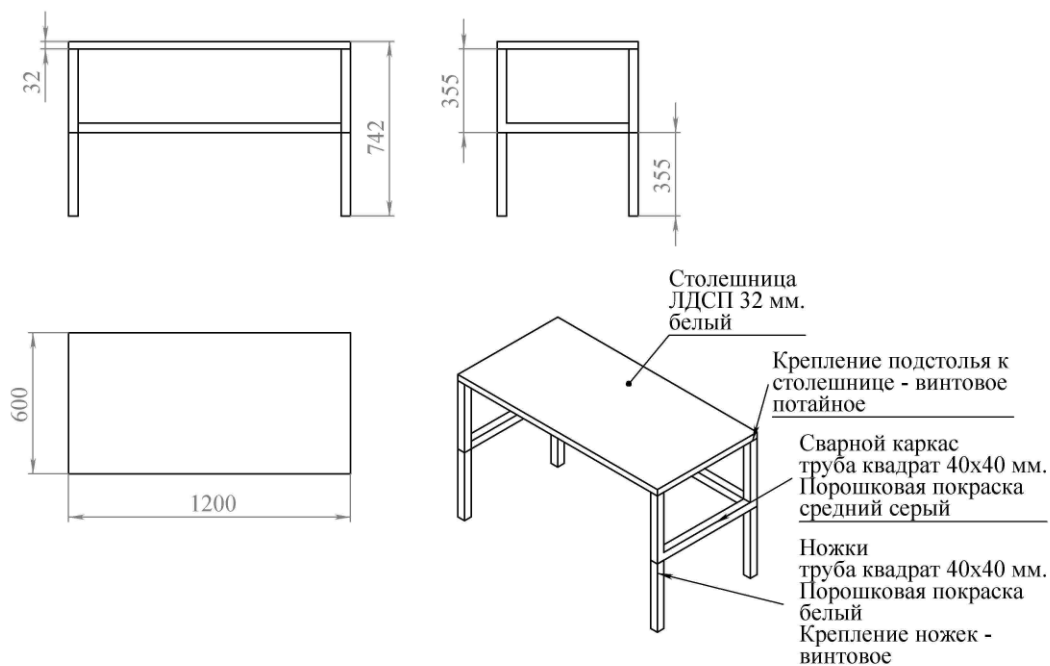
Стол ученический на сварном составном каркасном подстоле
