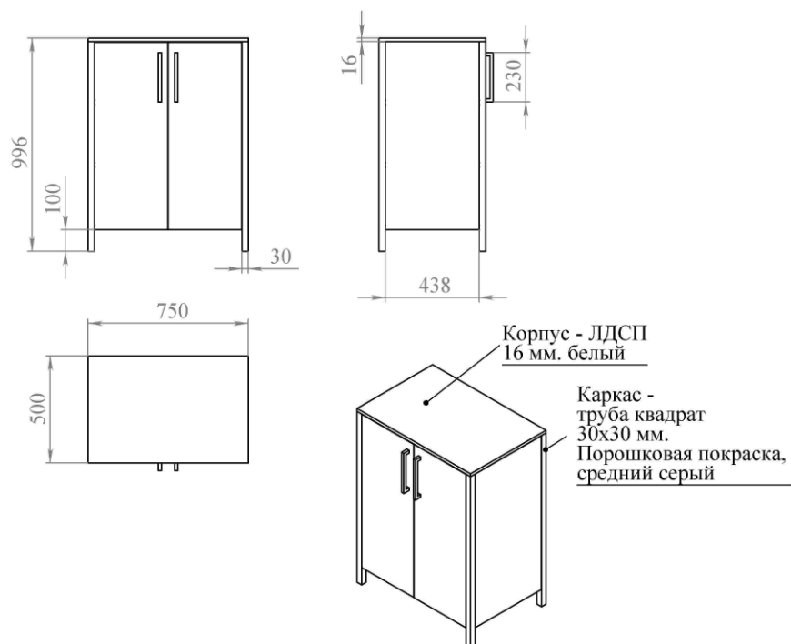
Тумба на сварном каркасе
